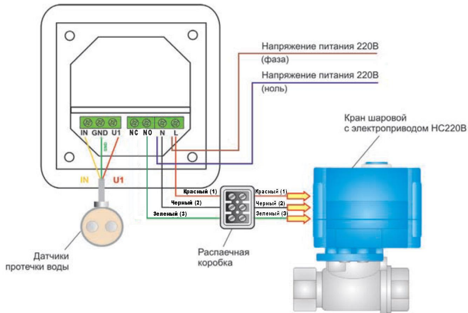
Схема подключения крана шарового с электроприводом HC к контроллеру SKPB220V-мини2N системы защиты от протечек "Нептун"
